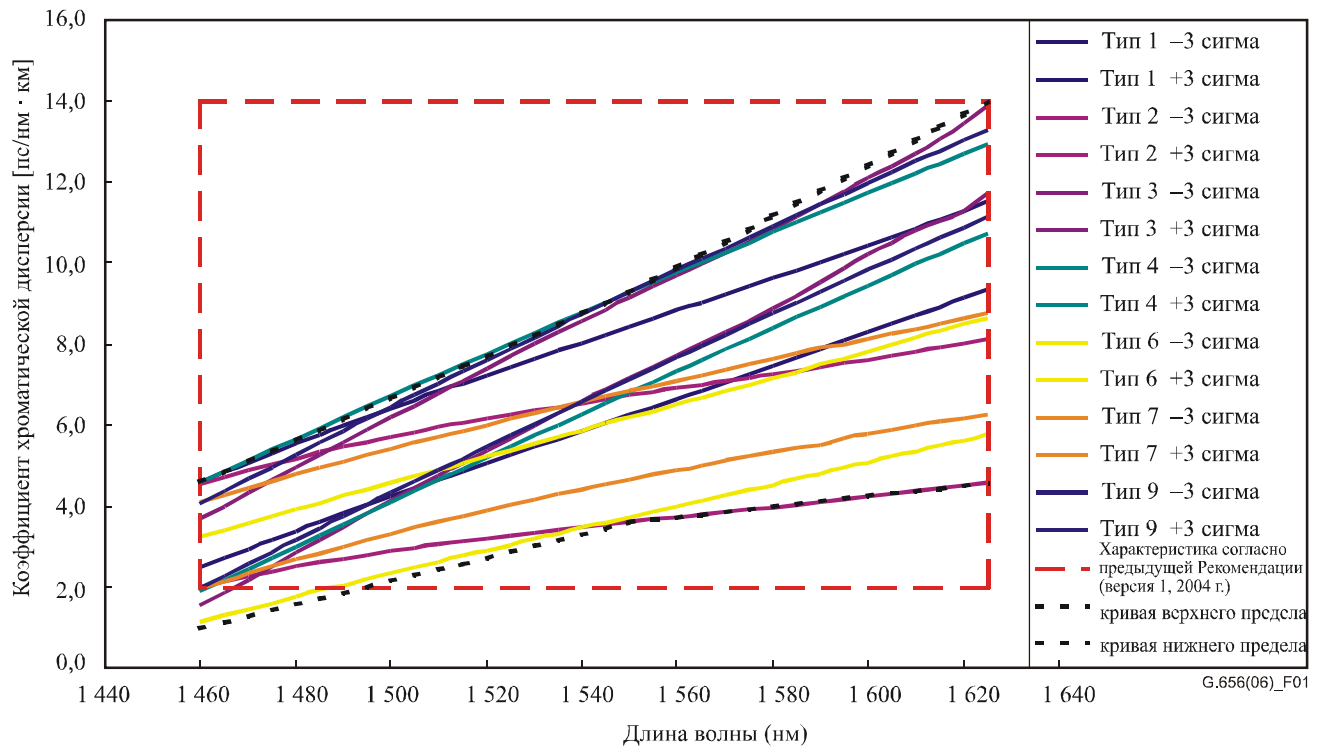
Рисунок I.1/G.656 – Дисперсия волокна, соответствующего данным таблицы 1
